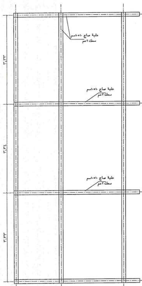
نموذج المظلة
