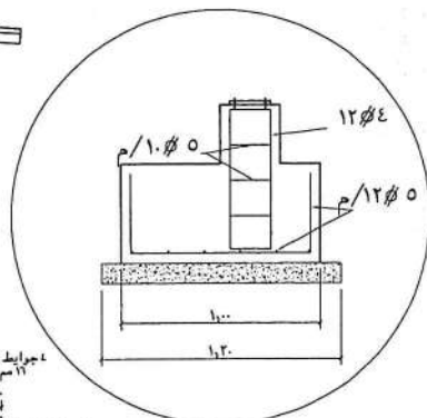
تفصيلة القاعدة
